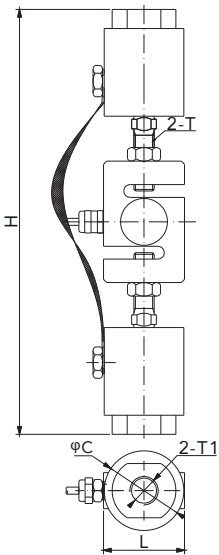
DIMENSIONS
